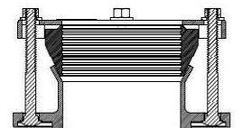
Brida según norma ISO7005-2
