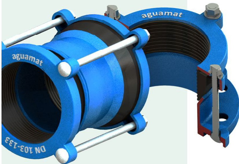
PERFORADO DE LA BRIDA SEGÚN NORMA ISO7005/2
